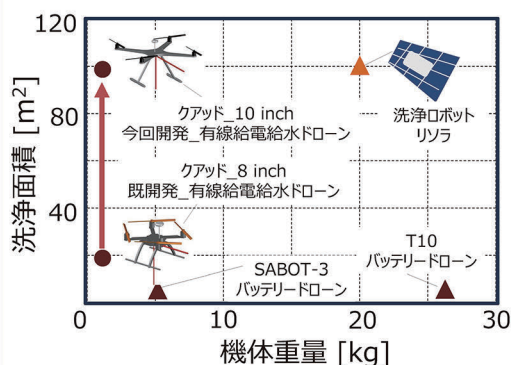
図1. 機体重量と洗浄面積の関係
