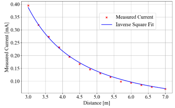
図5 光強度測定とフィッティング (距離減衰)
