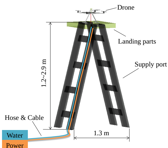
図 8 供給ポートと離着陸部に乗るドローンの概要図
