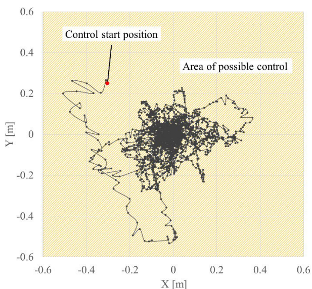
図 12 AR マーカー位置推定システム制御によるドローンの軌跡
