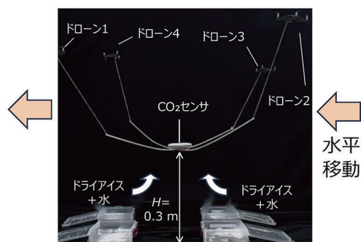
図4. ドローン4台によるCO 2 検知実験 (発生源直上10秒ホバリング)
