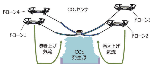
図3. ドローン4台の「巻き上げ気流」によるCO 2 検知
