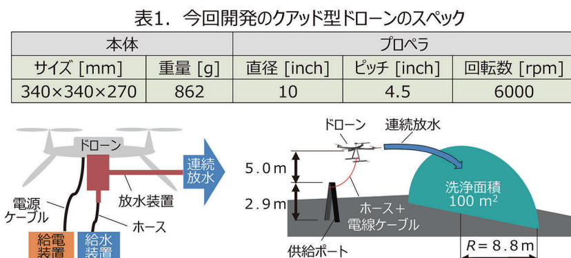
図2. 有線給電給水装置の概要
