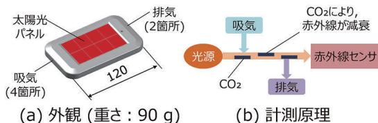
図2. 軽量のCO 2 センサ (RICOH D101)
