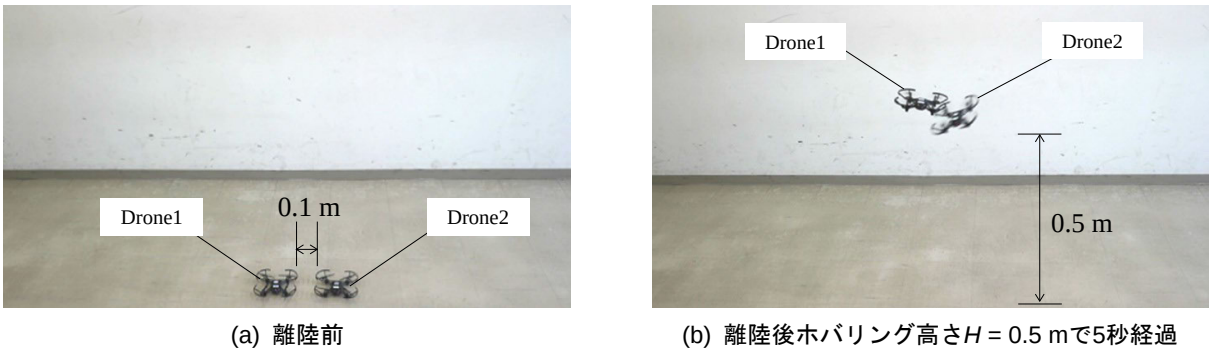
図 5 設置間隔 L=0.1 m の飛行実験 ( Re=0.5\times10^5 )
