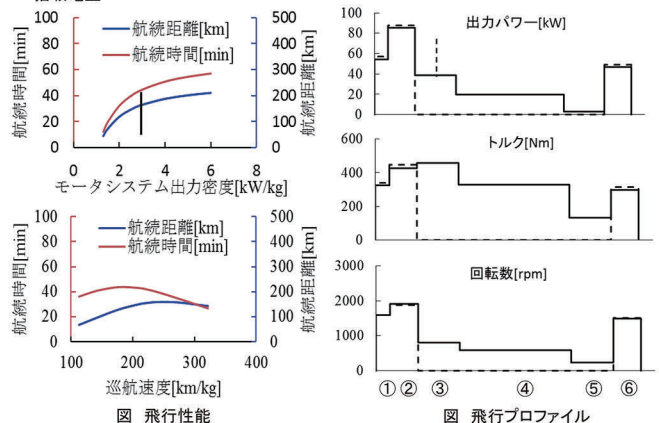
図 Wisk 社 eVTOL 機及び搭載したモータ (2022年10月公表)
