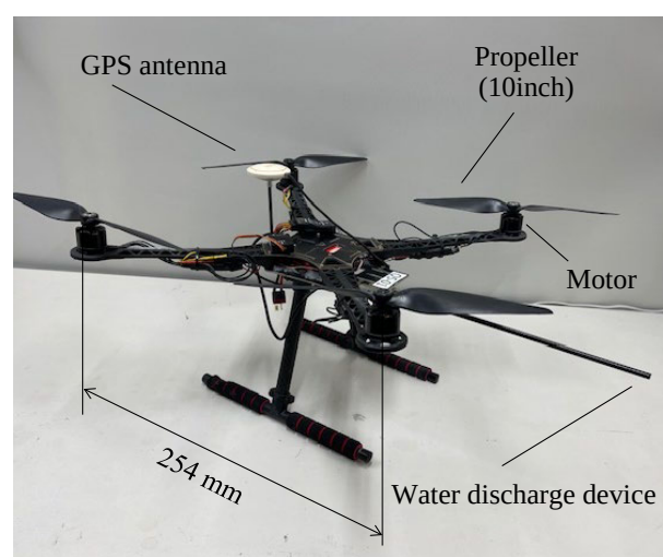
図 9 開発したドローンの写真
