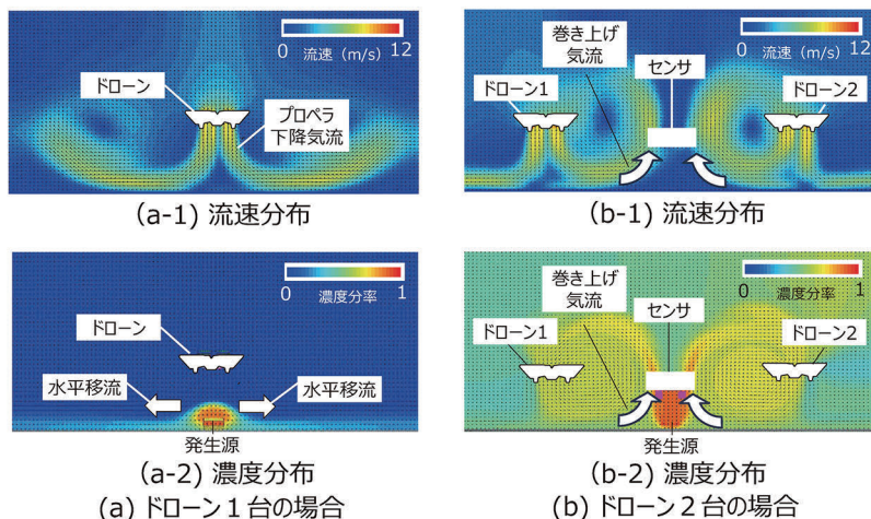
図1. ドローンまわりの流体シミュレーション
