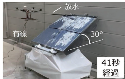
(a) 気流のみ (放水なし) による洗浄: 11秒 (b) 気流 + 放水による洗浄: 41秒 (c) 気流 + 放水による洗浄: 78秒
