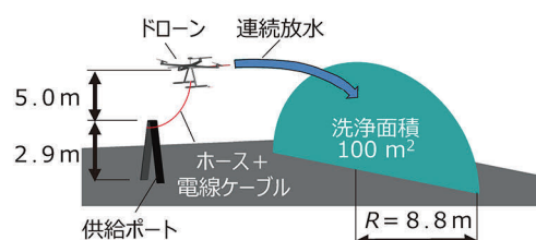
図3. 連続放水飛行の概略と放水面積
