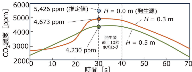
図5. 水平移動するドローンでのCO 2 検知実験における時系列濃度の結果
