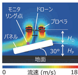
図4. 流体シミュレーション結果
