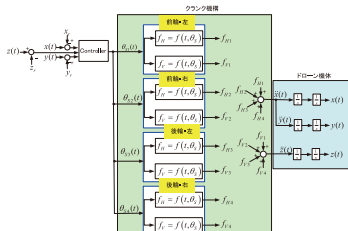
制御ブロック図
