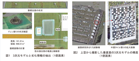
図1 3次元モデルと劣化情報の抽出(1億画素) 図2 上空から撮影した垂直面の3次元モデルの精度(1億画素)
